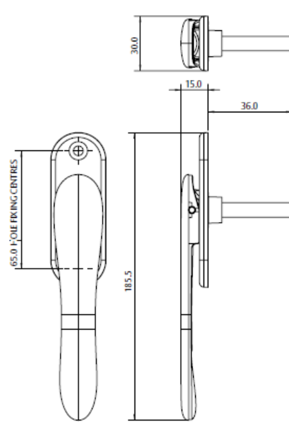
Uno Style Bi-fold Handle
